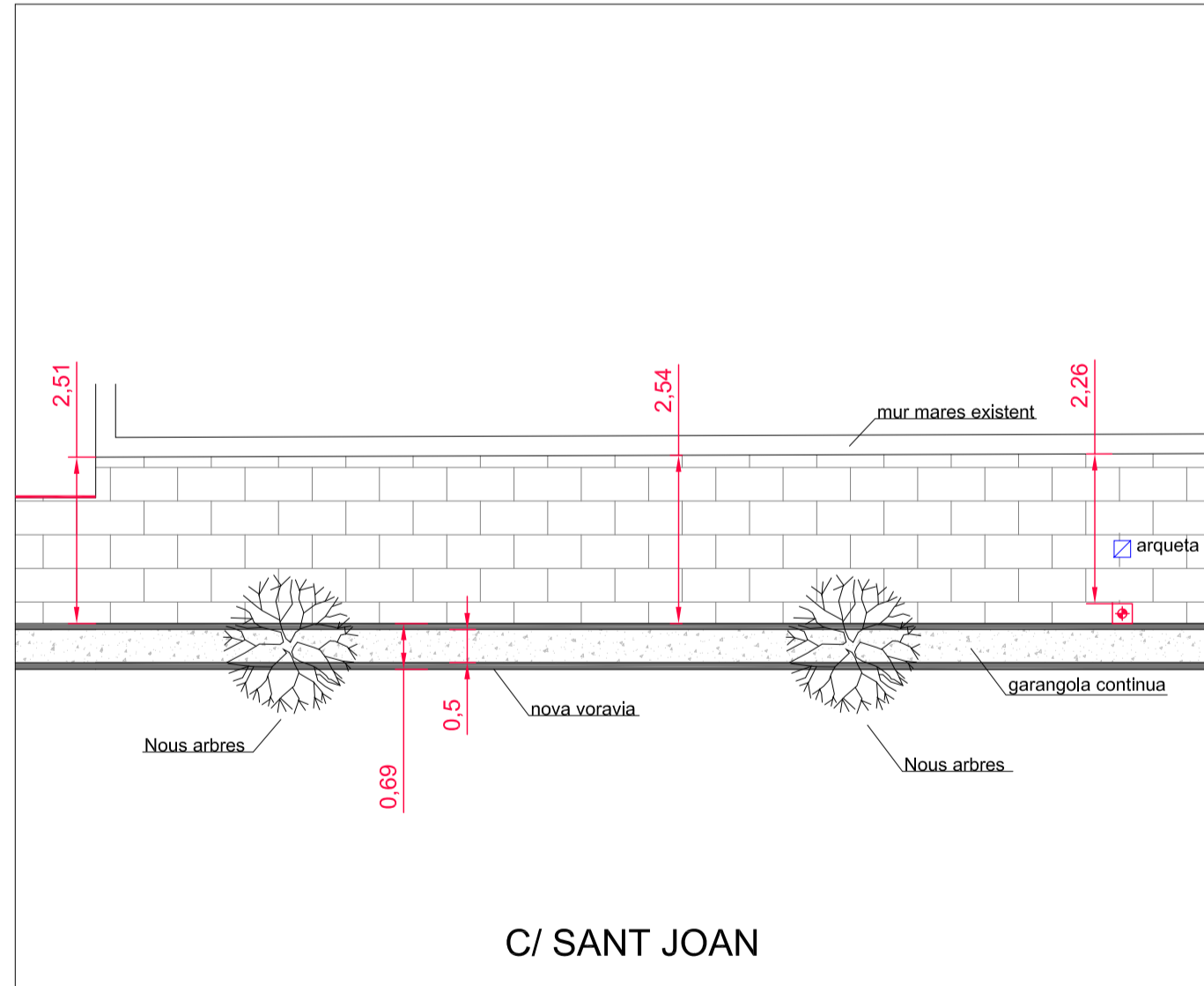
DETALL TRAM 2 (E 1/100)
